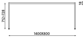
SIMPLE 140×80
